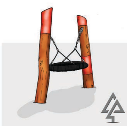
Mini Double Pole Basket Swing 222-MPS
